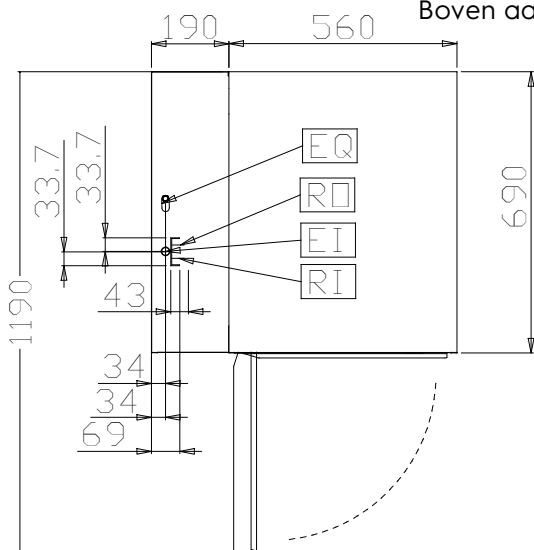
Boven aanzicht
