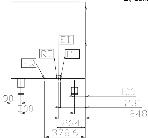
Zij aanzicht
